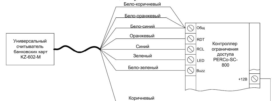
Рис.6. Схема подключения считывателя KZ-602-M к контроллеру ограничения доступа PERCo-SC-800
